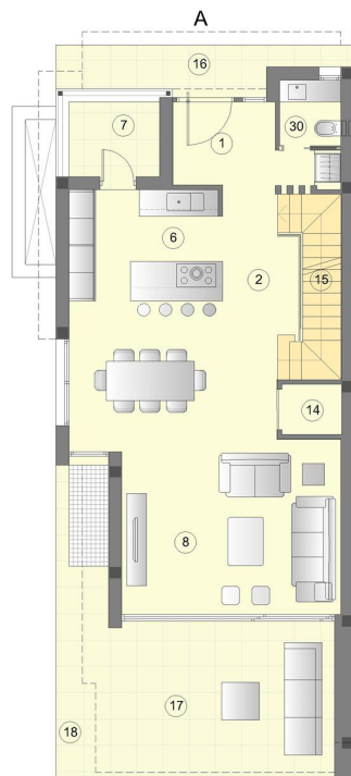
PLANTA BAJA
