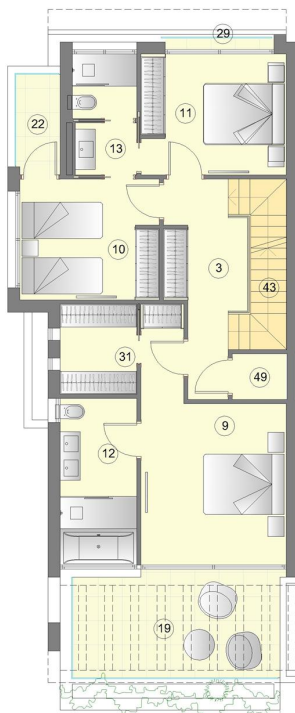
PLANTA PRIMERA
