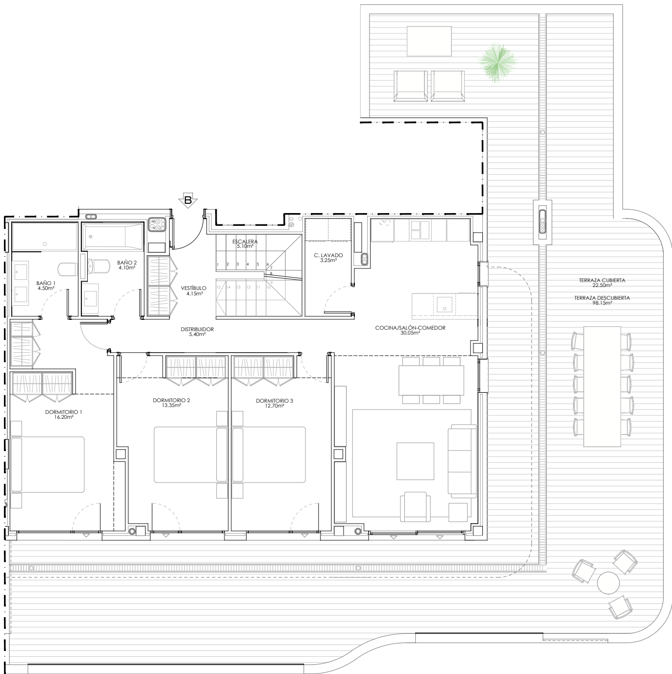
PL. SEGUNDA
