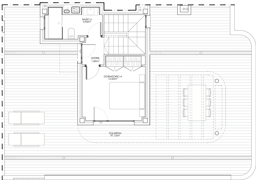
PL. ÁTICO
