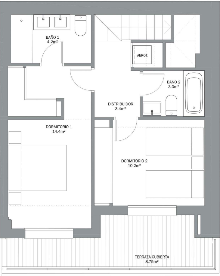
PLANTA DORMITORIOS
