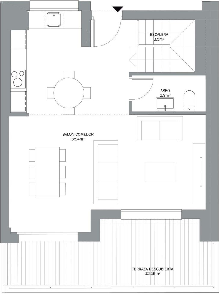
PLANTA ACCESO
