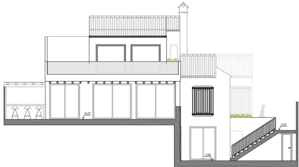
SECCION S3
