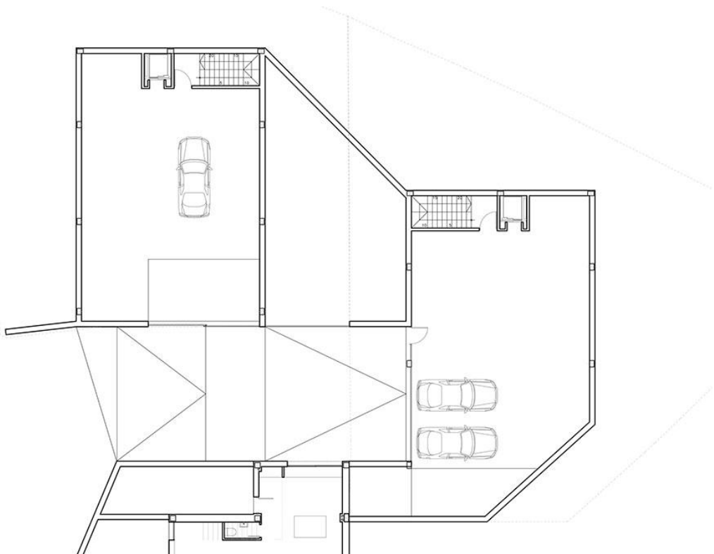
PLANTA SOTANO
