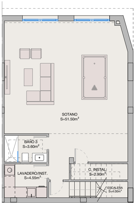
planta sotano
